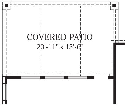
OPTIONAL EXTENDED PATIO
