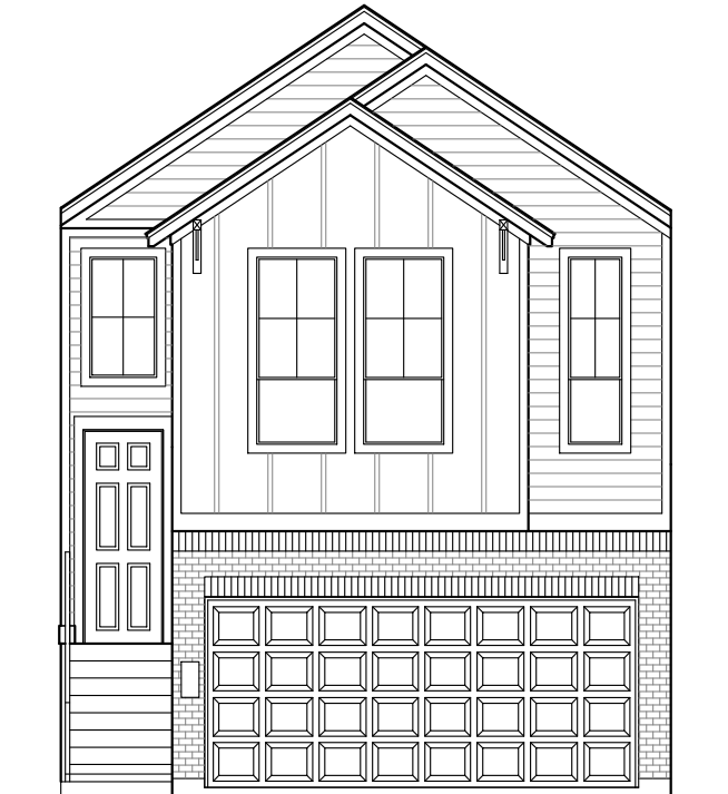
ELEVATION B
