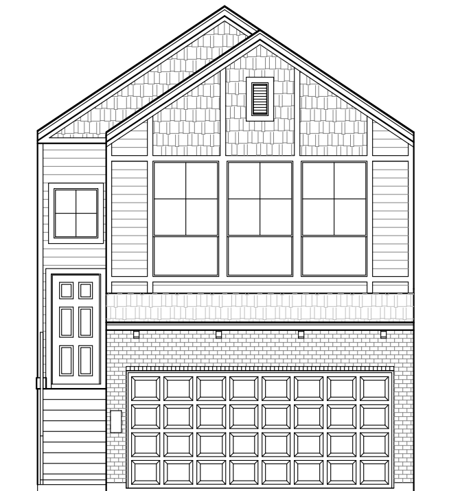
ELEVATION B
