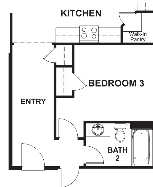
OPT. BEDROOM 3
