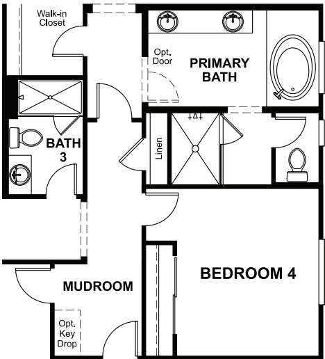
OPT. BEDROOM 4/BATH 3
