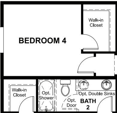
OPT. BEDROOM 4
